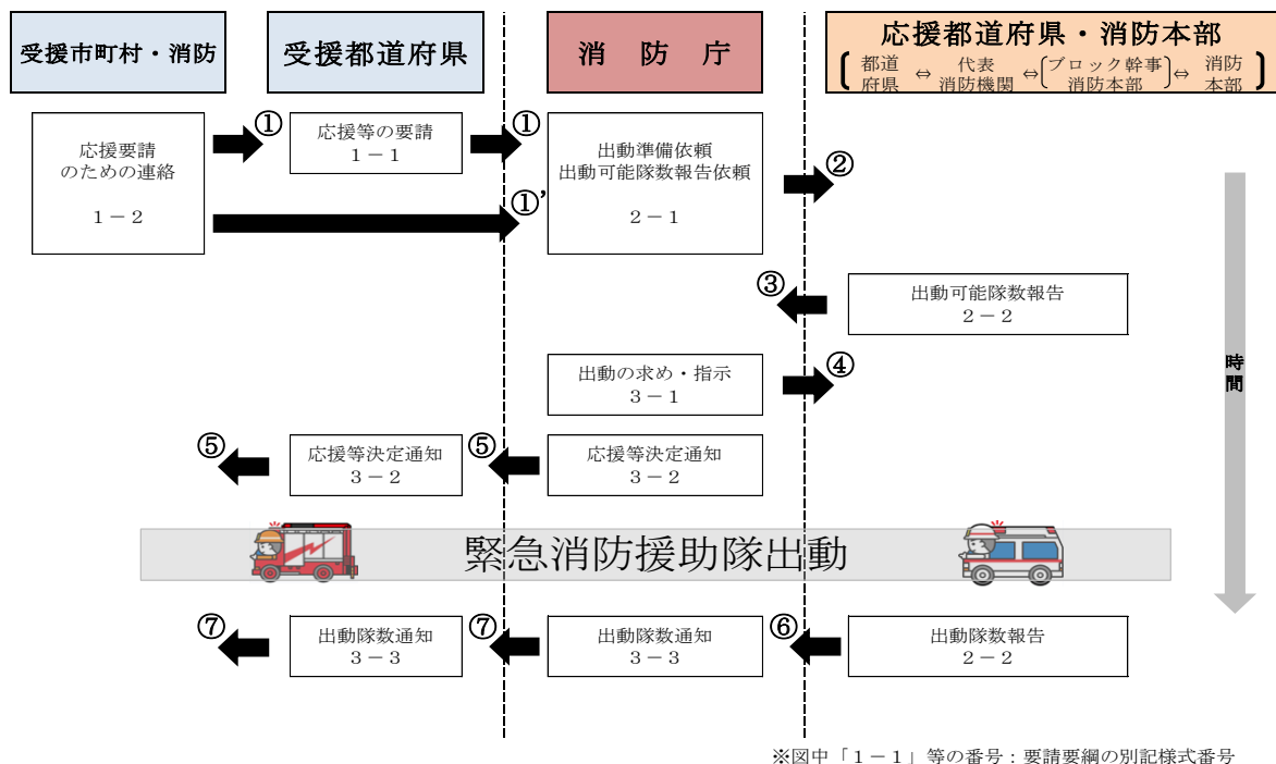
別図第1 緊急消防援助隊 応援要請系統図
