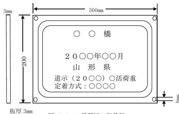
図 12-4-1 橋歴板の記載例
