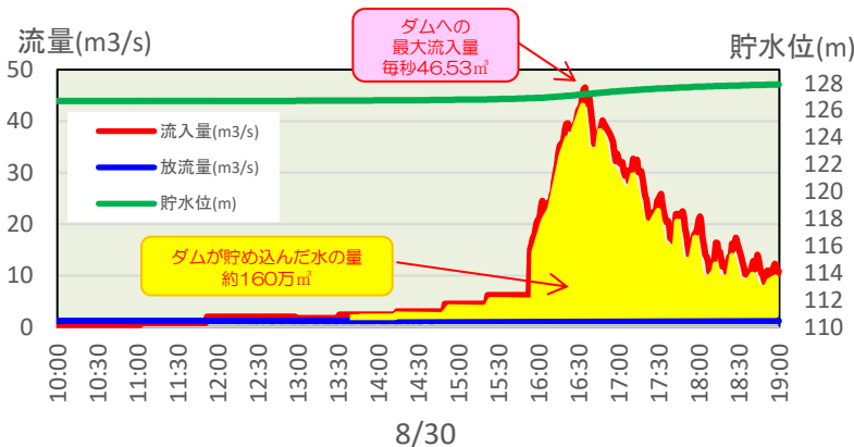
ダム流入量/放流量/貯水位
