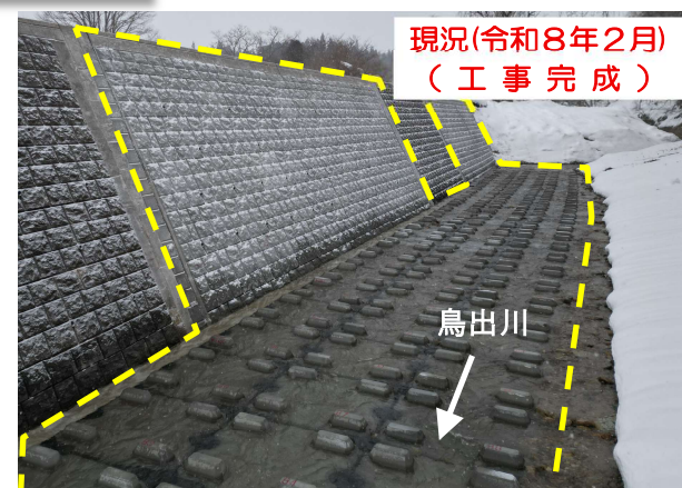
崩れた護岸をコンクリートブロックで復旧しました
