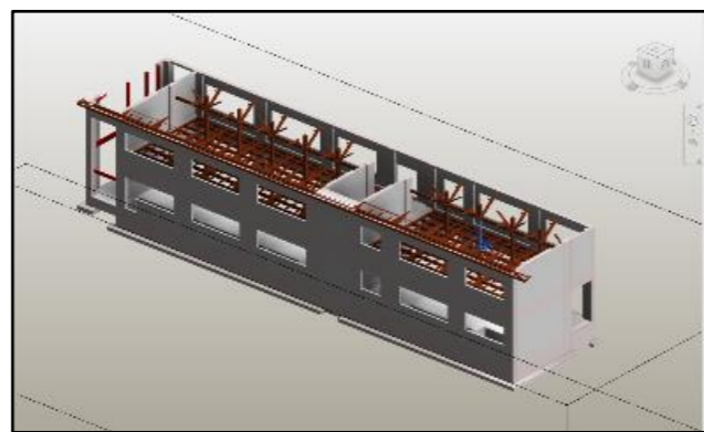
BIMモデル（構造）
